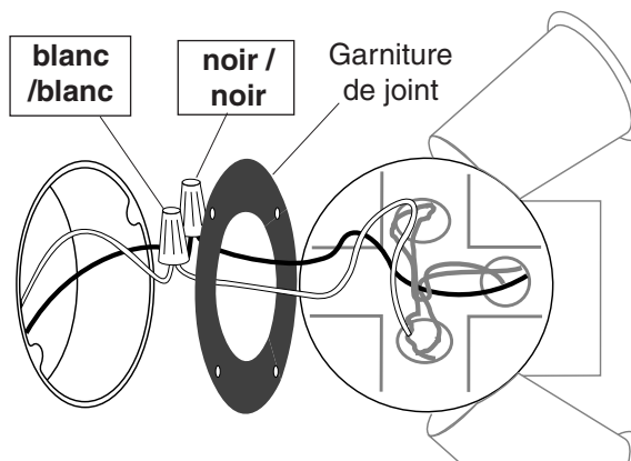
Montage mural
